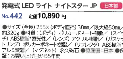
発電式LEDライト ナイトスター JP 日本製 No.442 定価10,890円 ●サイズ: (全長) 255×(ボディ直径) 38mm/最大径50mm/約320g ●材質: (ボディ) ポリカーボネート樹脂/ (スイッチ) ABS樹脂*蓄光性/ (レンズ) アクリル樹脂/ (ガasketリング) ポリカーボネート樹脂/ (リフレクタ) ABS樹脂*アルミ蒸着/ (マグネット) 永久磁石 ●原産国: 日本 ●保証: お買い上げ日から5年間
